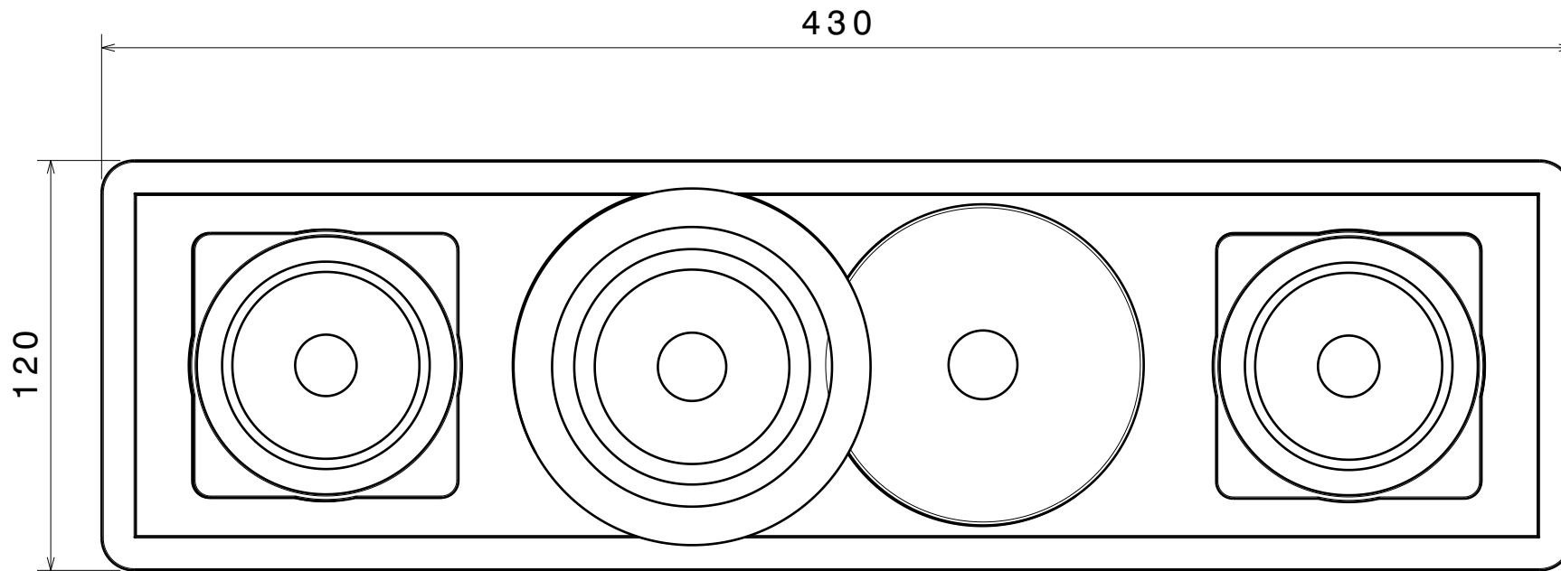
Vorderansicht Maßstab: 1:2
